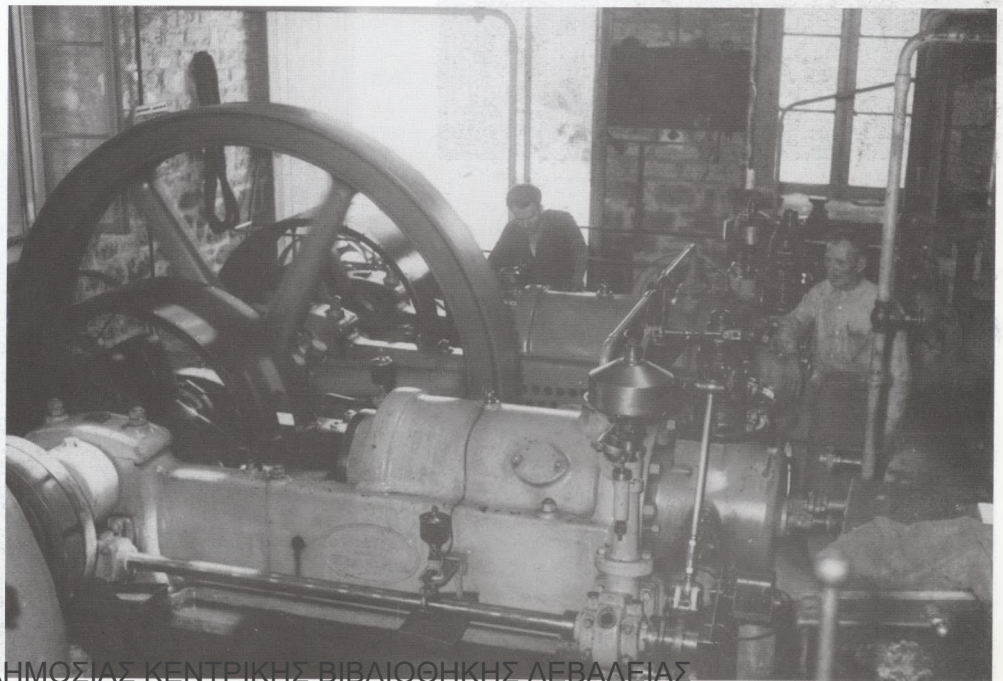
24. Η ηλεκτρογεννήτρια του σταθμού
