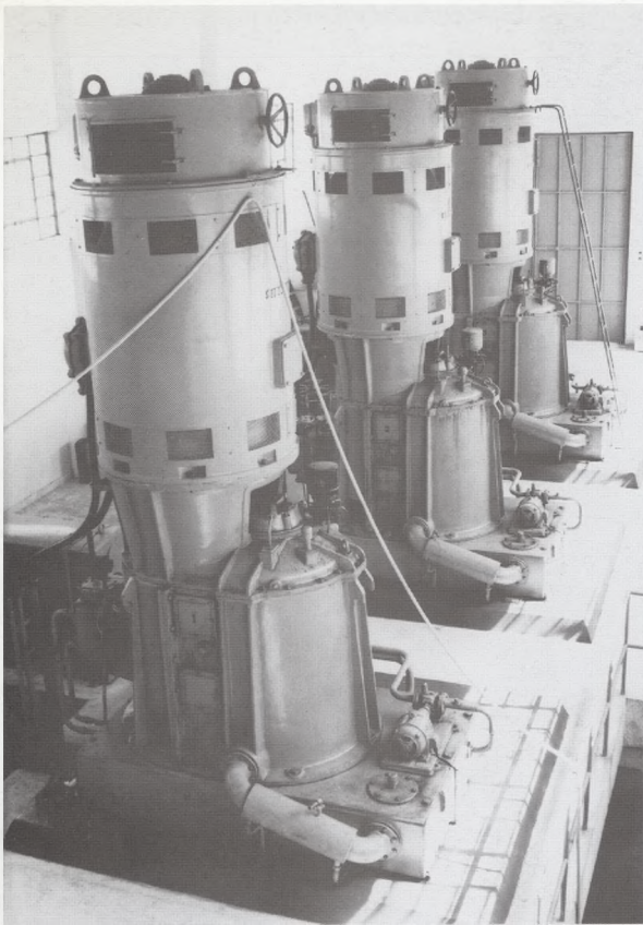
30. Η τεχνική υποδομή του νέου αντλιοστασίου της Γλίκης
