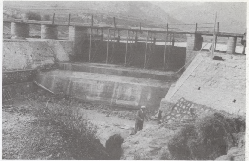
17. Κατασκευή κεντρικού υδατοφράκτη το μεσοπόλεμο
