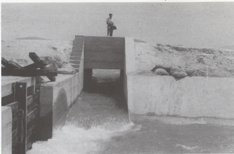
25. Τοπικοί διακλαδωτές καναλιών
